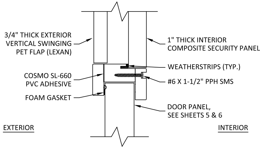
B 4 VERTICAL SECTION PET DOOR SILL
