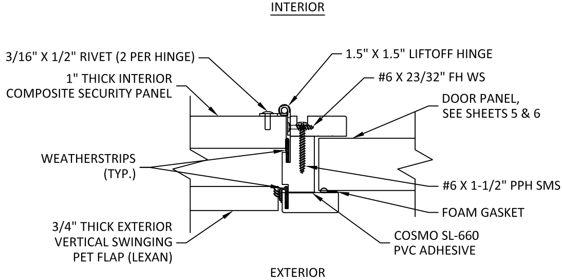
D 4 HORIZONTAL SECTION PET DOOR HINGE JAMB
